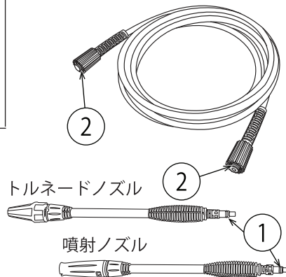
NJC110-10M用高圧ホース
