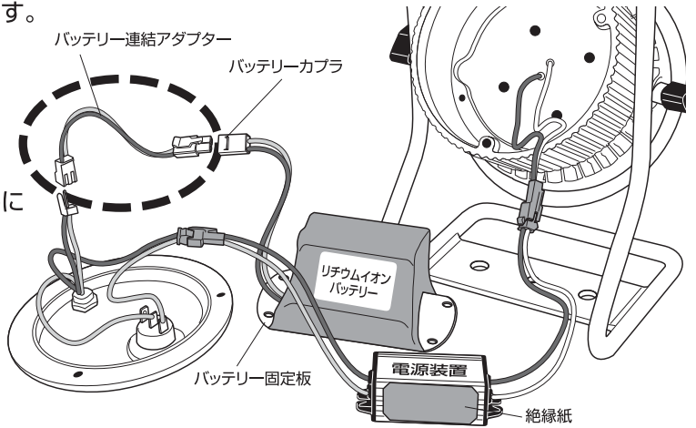
組立て図
