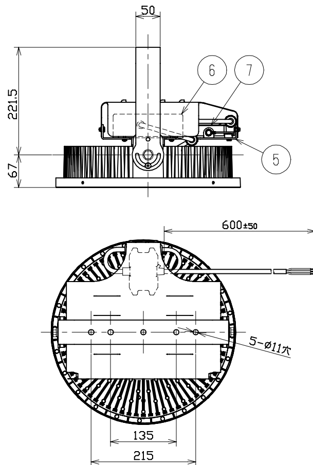
A矢視図
